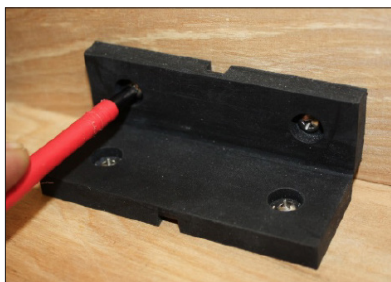
Immagine #1. Fissaggio dell'AV Pad in posizione angolare
